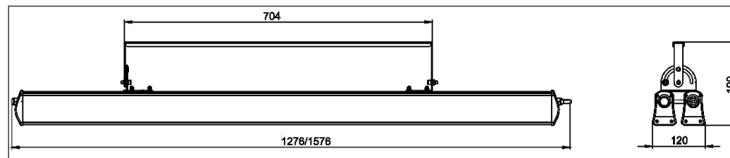
Габаритные размеры светильника
