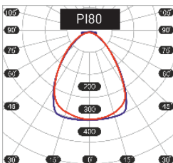
Диаграмма силы света
