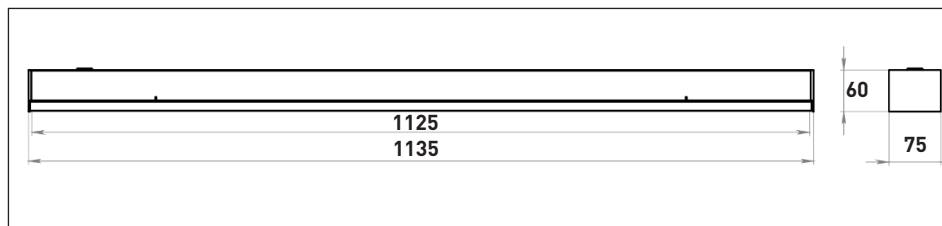
Габаритные размеры светильника
